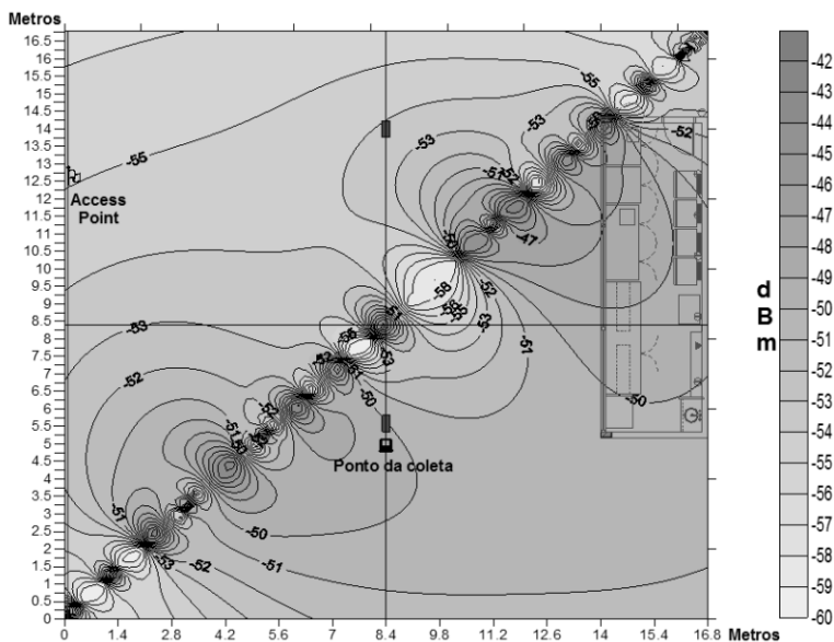
Figura 3 - Análise do sinal wireless no setor de vivência realizando download .
