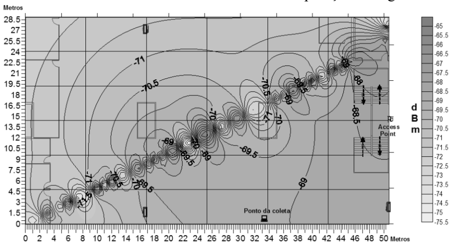
Figura 2 - Análise do sinal wireless na biblioteca Cor Jesu sem a realização do download .
