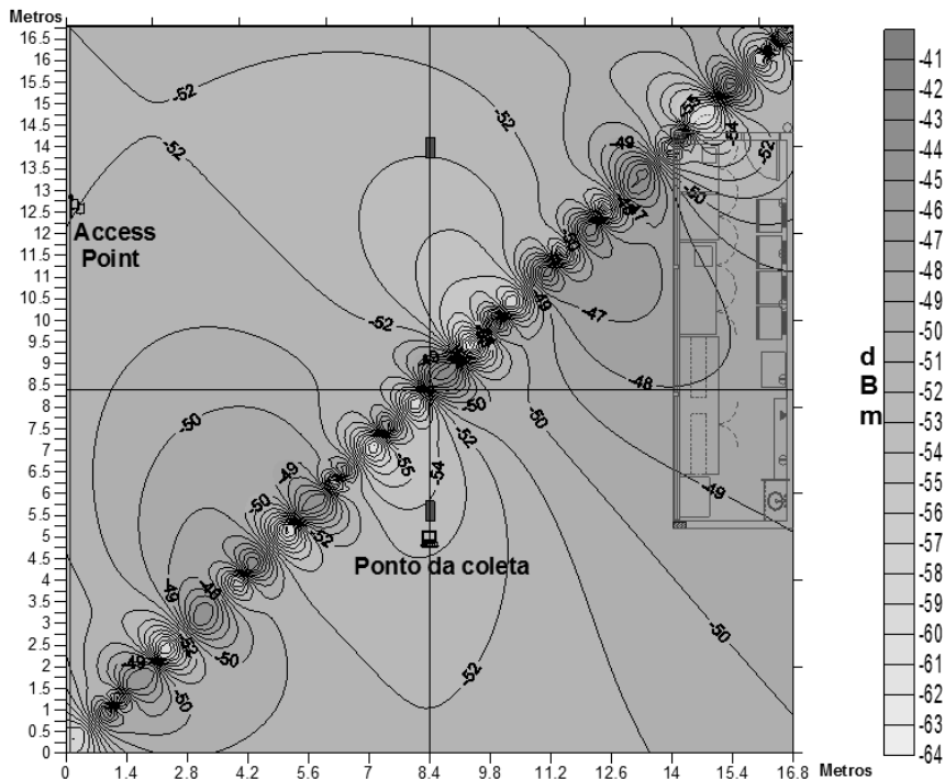
Figura 4 - Análise do sinal wireless no setor de vivência sem a realização do download .
